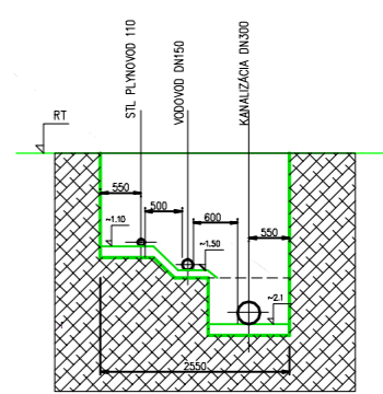
obrázok: typová schéma uloženia technickej infraštruktúry
